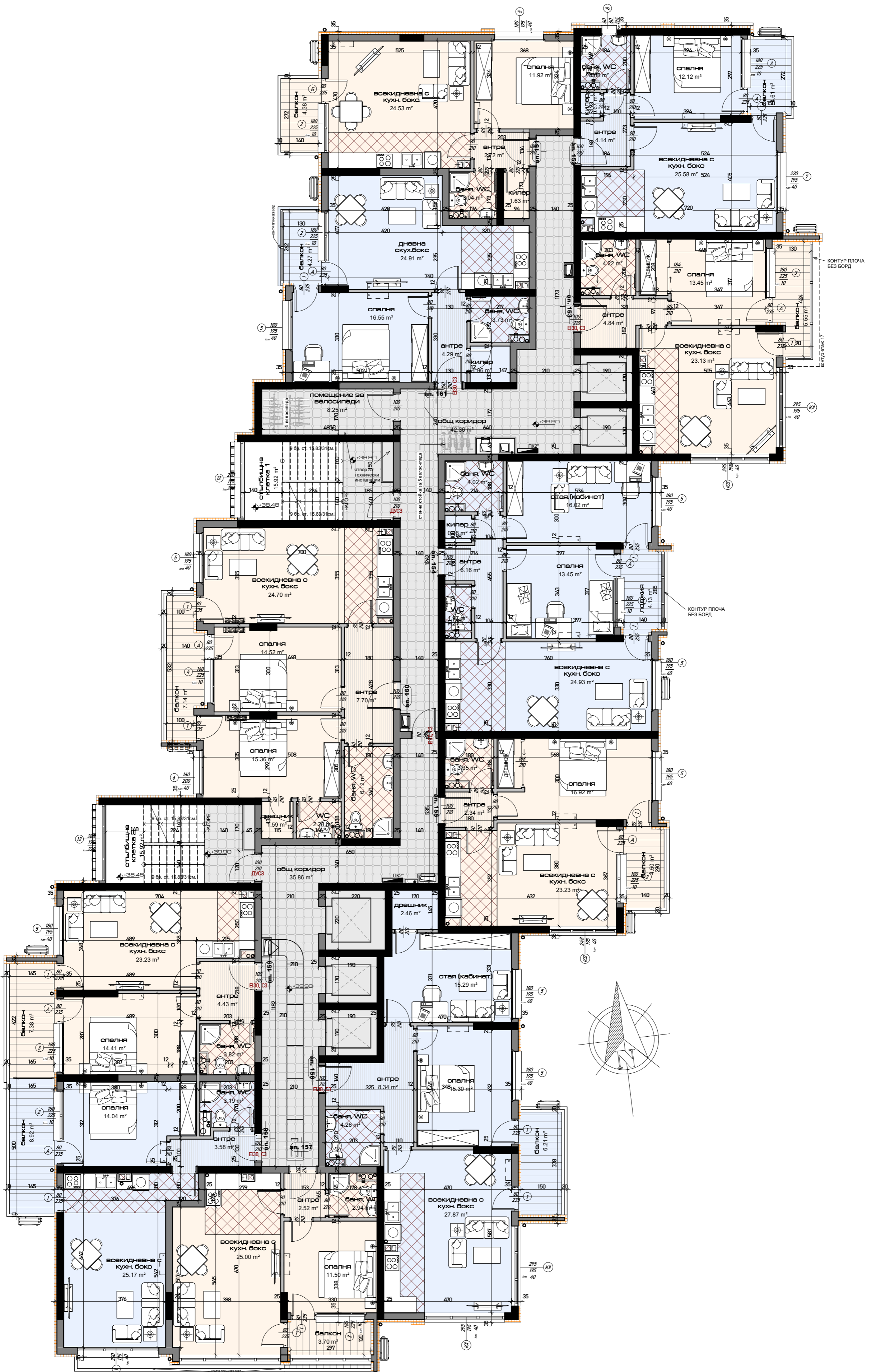
21 РАЗПРЕДЕЛЕНИЕ ЕТАЖ 16 (к.т. +39.90м.) мащаб 1:100
